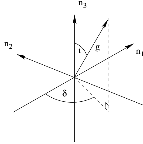
Figure 4: The gnomon.
